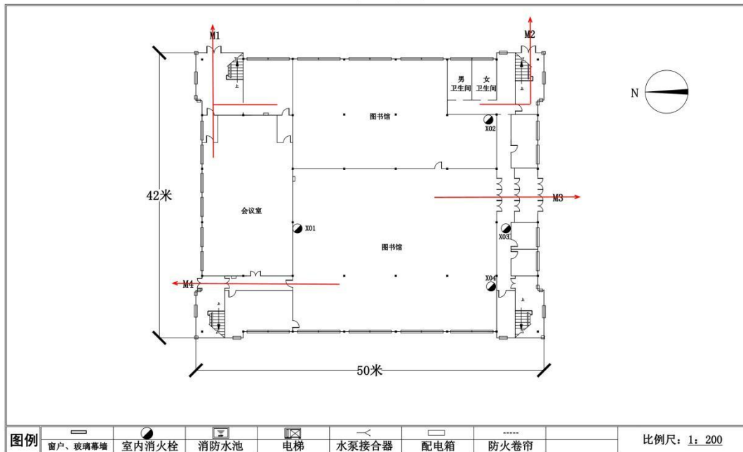
( 一 ) 层平面指挥图
