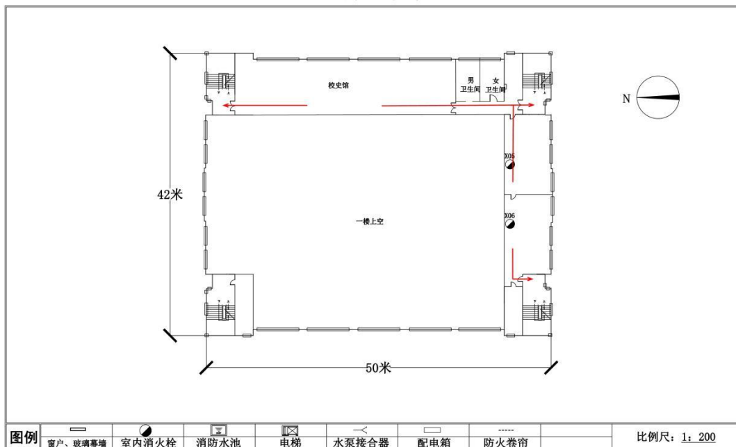
( 二 ) 层平面指挥图
