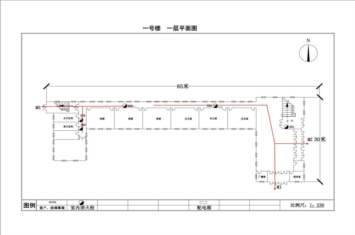
一号楼疏散图
