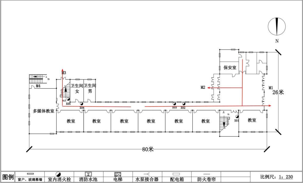
二号楼 一层平面图
