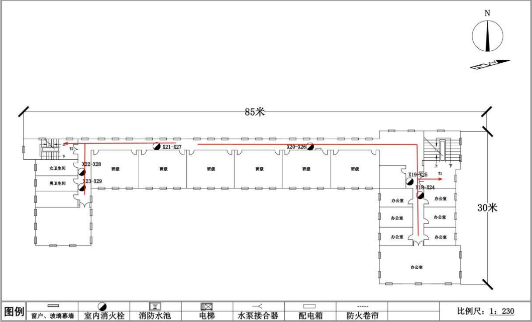
一号楼 四至五层平面图
