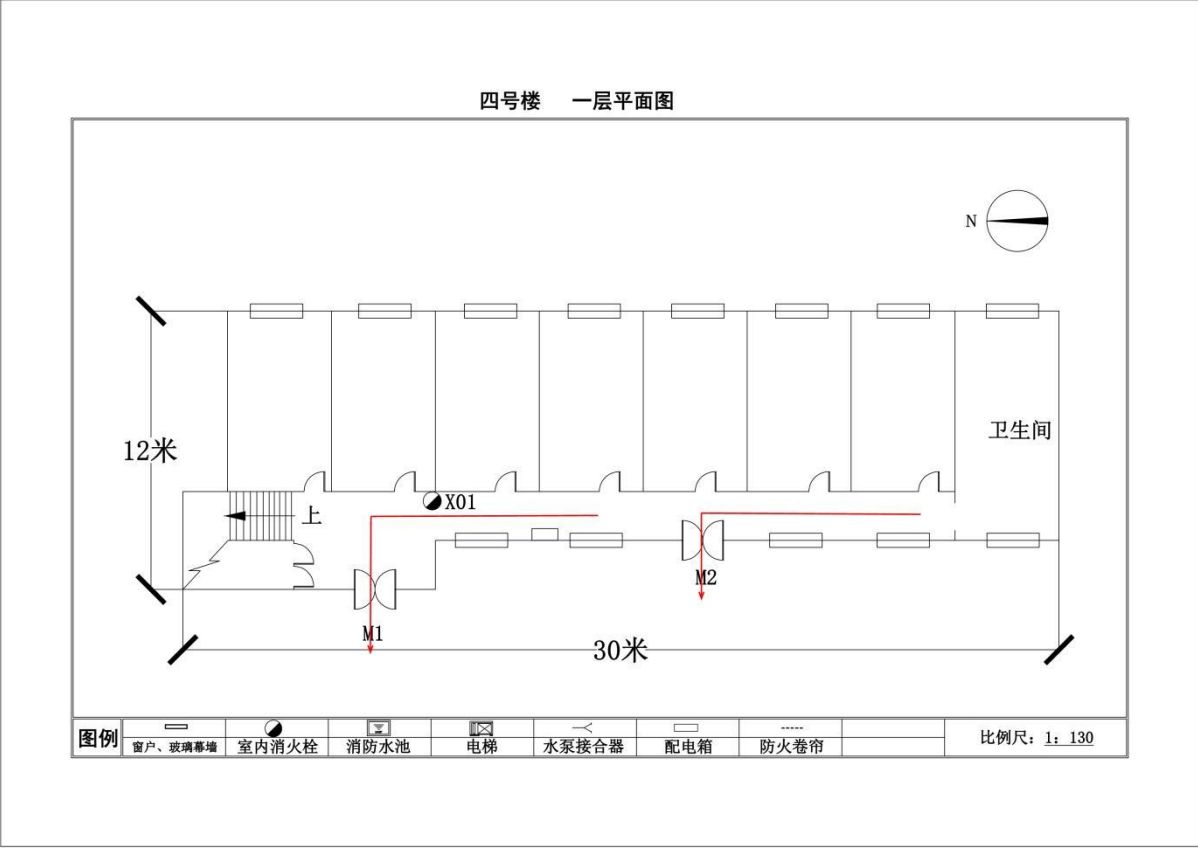
四号楼疏散图
