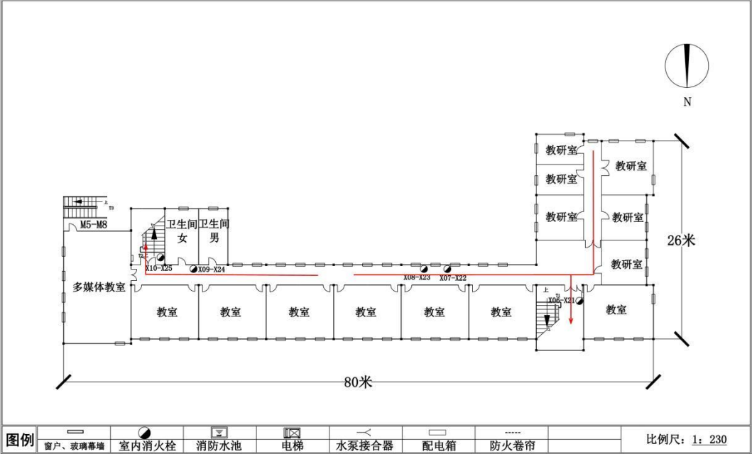
二号楼 二至五层平面图
