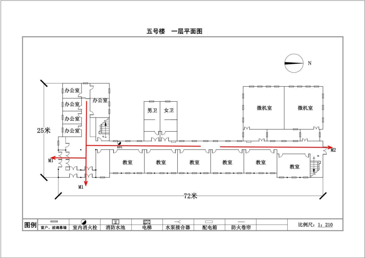
五号楼疏散图
