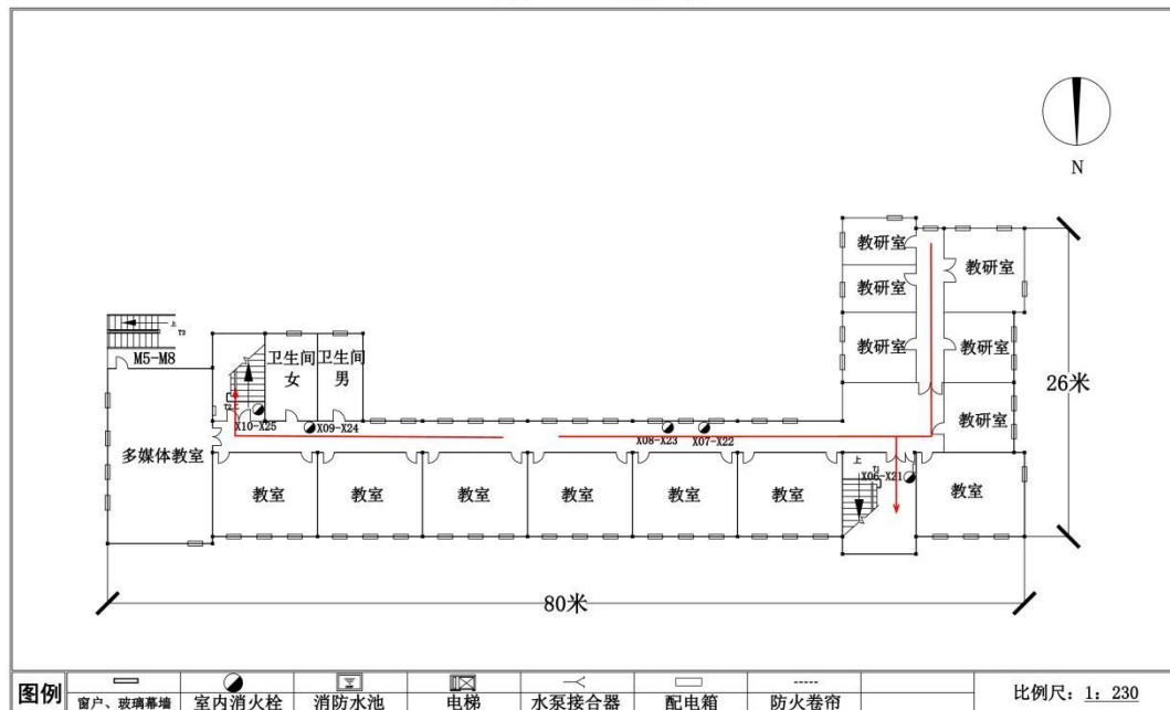
二号楼 二至五层平面图
