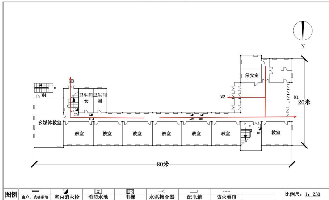
二号楼 一层平面图
