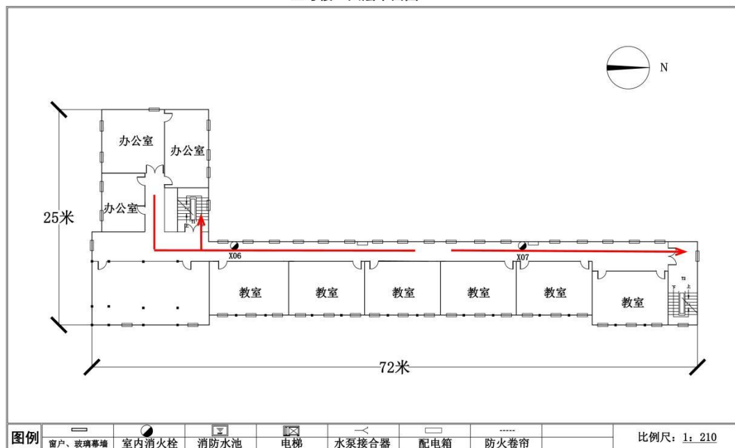
五号楼 四层平面图
