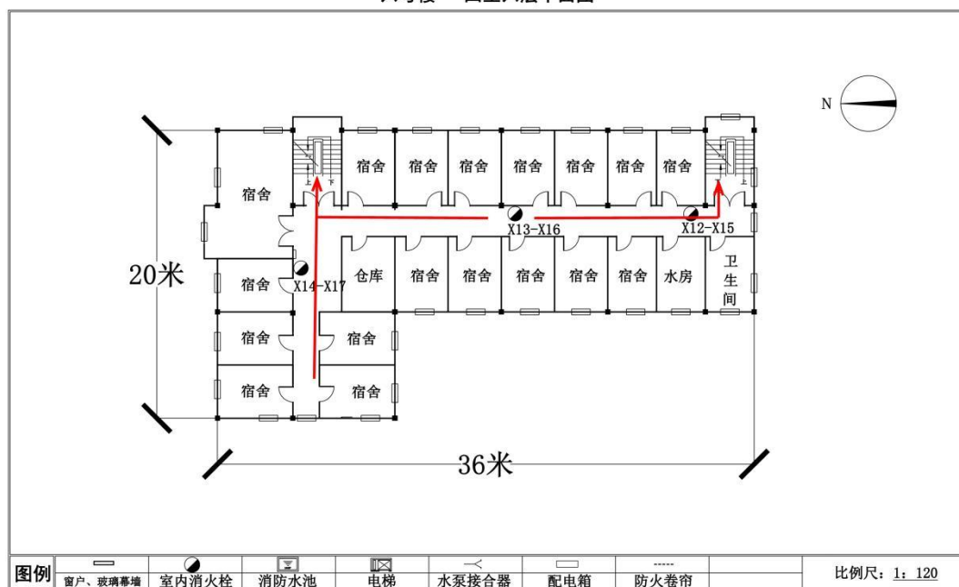
六号楼 四至六层平面图
