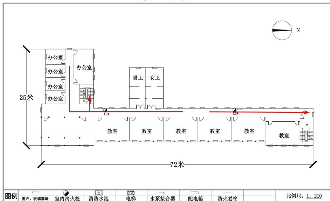
五号楼 三层平面图
